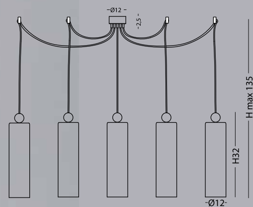
Tamigi S5 multicolor Vetro liscio Ø 12_H max 135_5-E27
