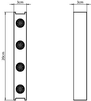
BLOKINLINE MODULE 4
