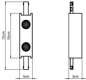
BLOKINLINE MODULE 2
